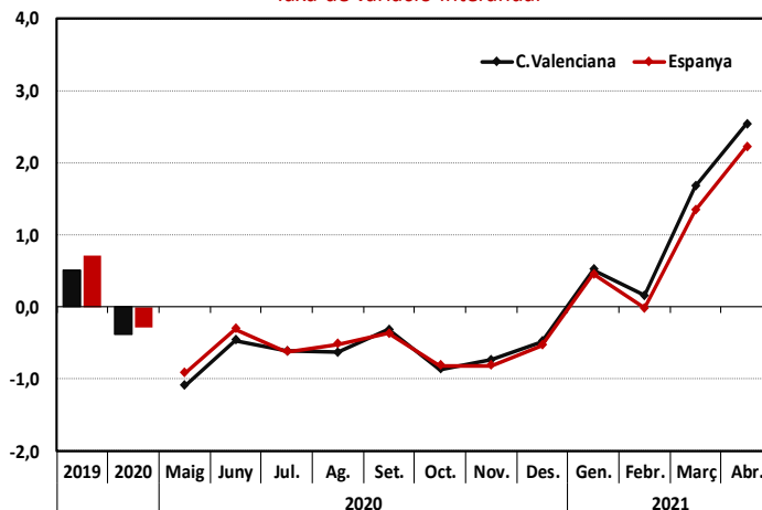
Índice de preus de consum Taxa de variació interanual
