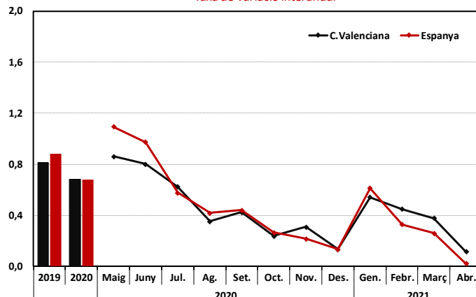
Índice de preus de consum sense aliments ni energia Inflació subyacent Taxa de variació interanual
