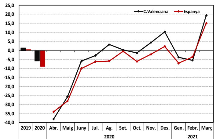
Índice general de producción industrial Taxa de variació interanual
