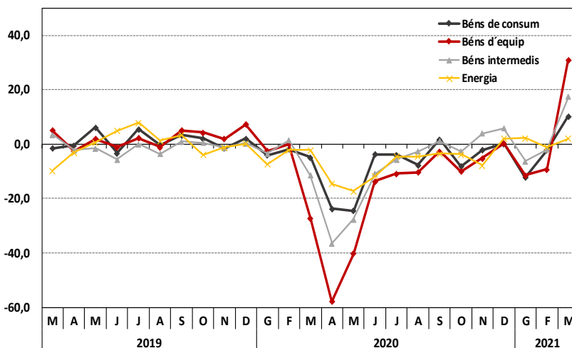
Índice general de producción industrial per destí econòmic dels béns Espanya Variació interanual (%)
